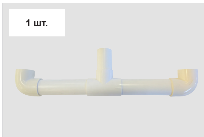
Трубопровод вакуумный (комплект)
